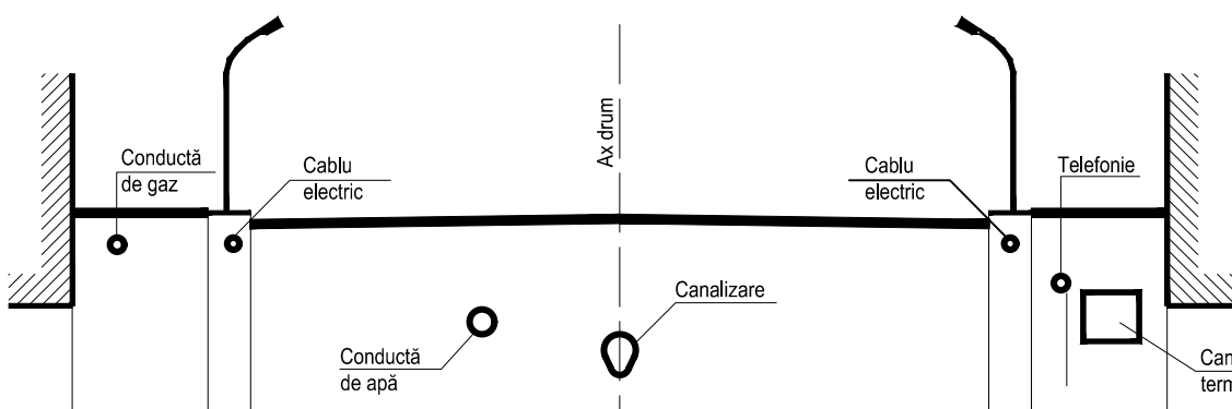
EXEMPLU AMPLASAREA ÎN LOCALITĂȚI A REȚELOR EDILITARE SUBTERANE, EXECUTATE ÎN SĂPĂTURĂ
